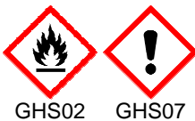
GHS02 GHS07
